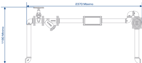
DIMENSÕES PRINCIPAIS (mm)
