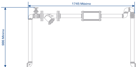
DIMENSÕES PRINCIPAIS (mm)
